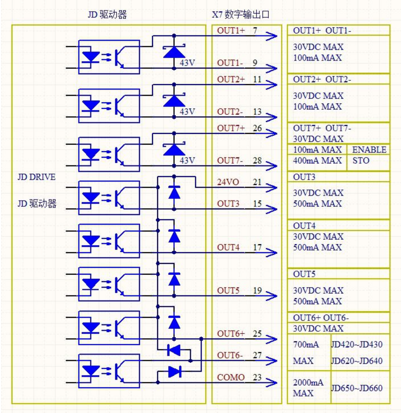
图 7-6 数字输出口内部电路图
