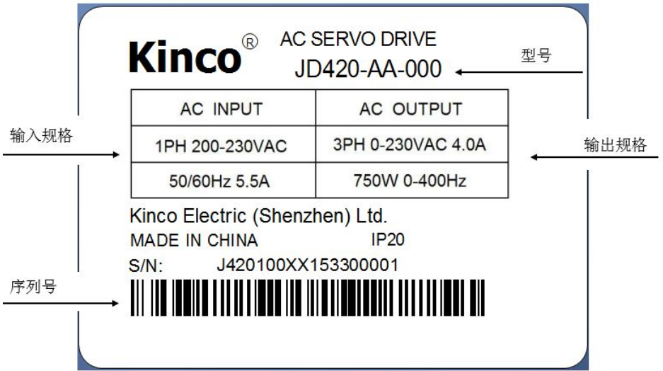
图 1-1 伺服驱动器铭牌
