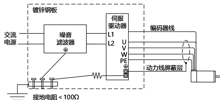
图 3-6 滤波器连接示意
