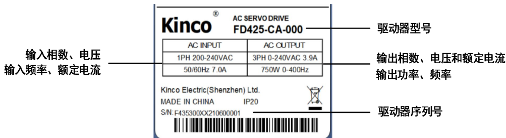
图 1-2 驱动器铭牌说明
