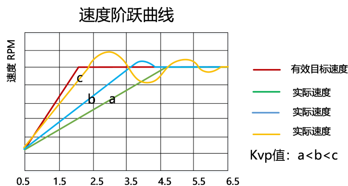
图 7-4 速度环比例增益调节后的速度阶跃曲线
