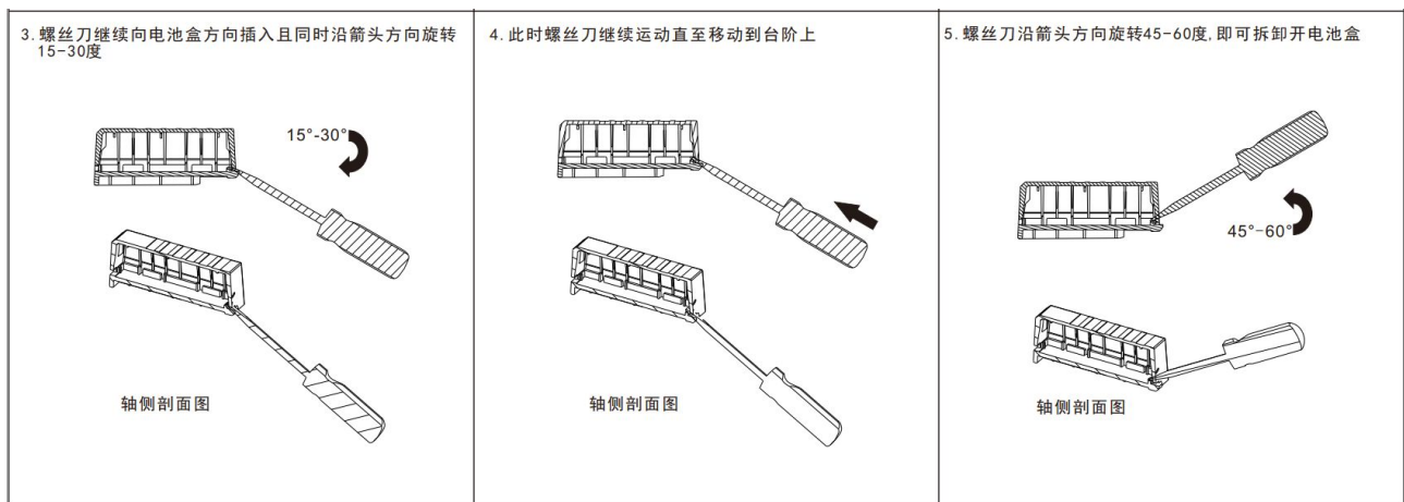
图 6-13 电池盒拆卸方式
