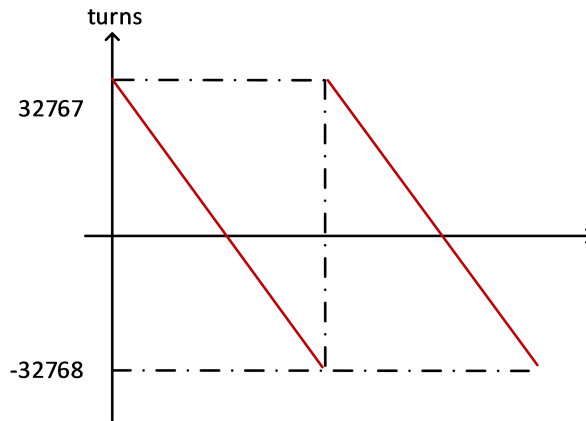
图 6-12 多圈数据范围
