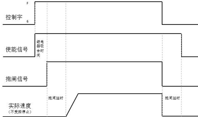
图 6-11 快速停止模式为 0 时电机抱闸时序
