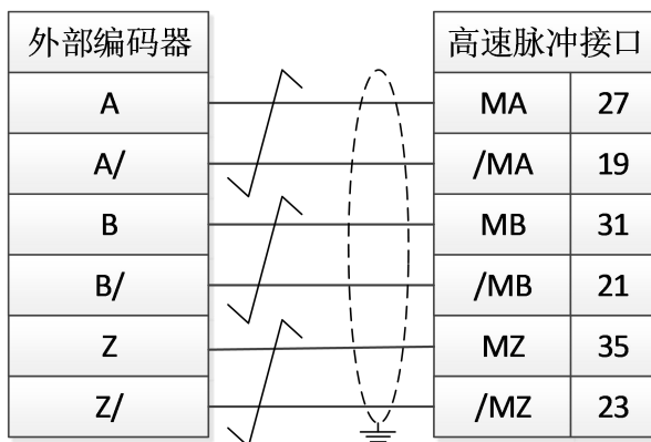
图 6-8 全闭环控制连接高速脉冲接口
