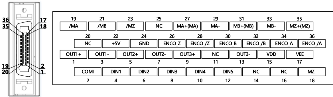
图 3-14 FD5-PA 驱动器外部输入输出端子引脚示意
