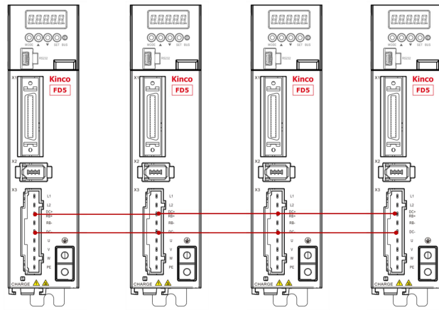
图 3-9 FD425 共直流母线
