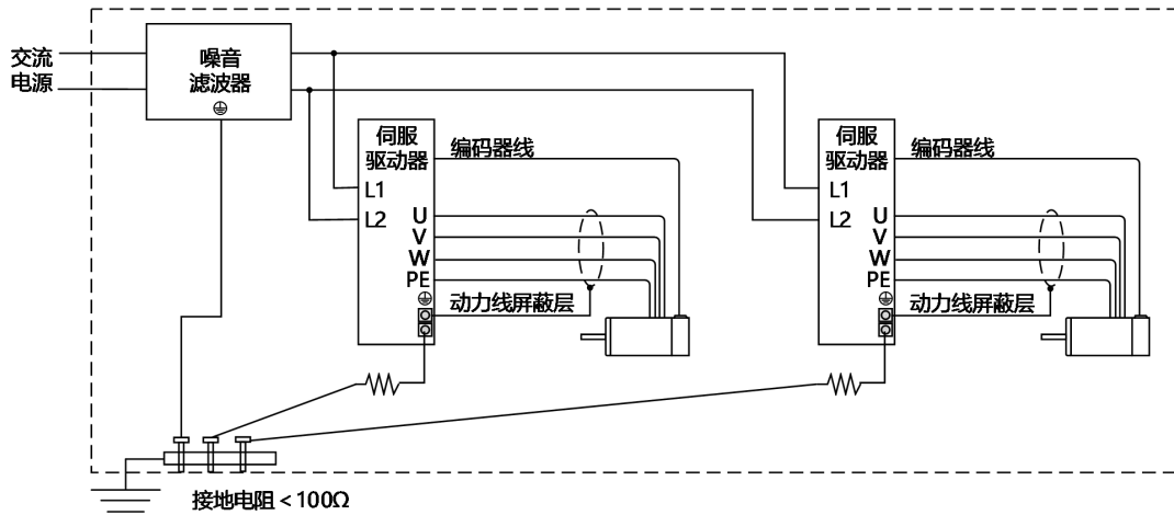
图 3-7 多台驱动器接地方式
