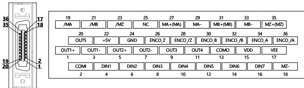
图 3-12 FD5-LA/CA 驱动器外部输入输出端子引脚示意
