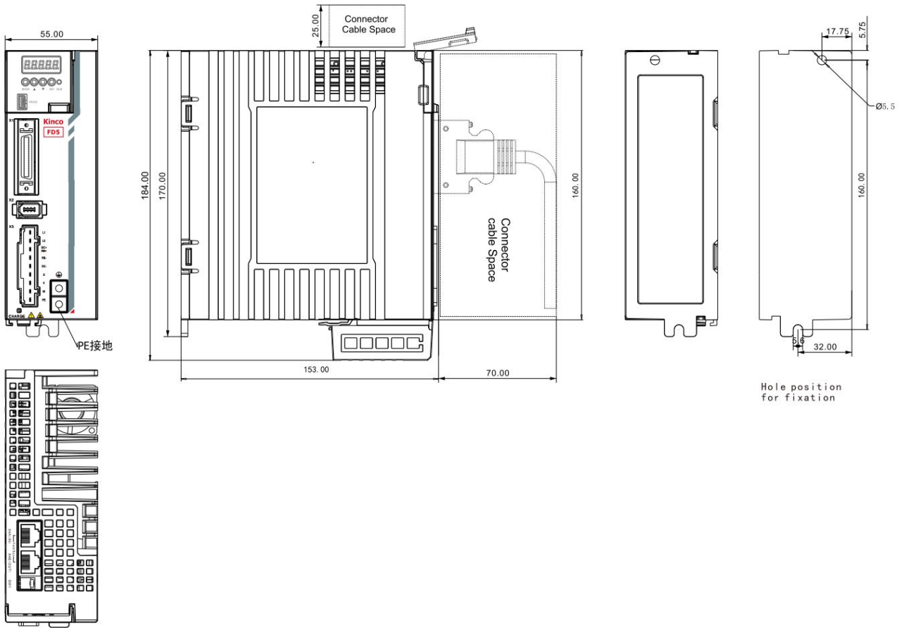
图 2-2 FD425-□F(1000W)产品安装图
