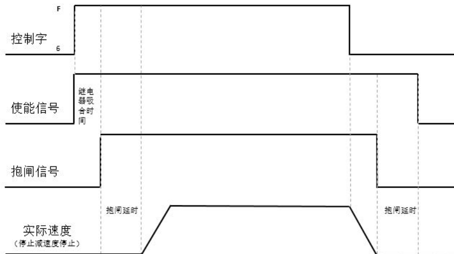
图 6-12 快速停止模式为 0 时电机抱闸时序
