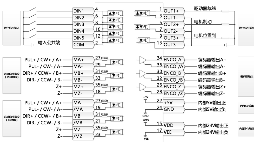
图 3-15 FD5-PA 驱动器 IO 口默认定义
