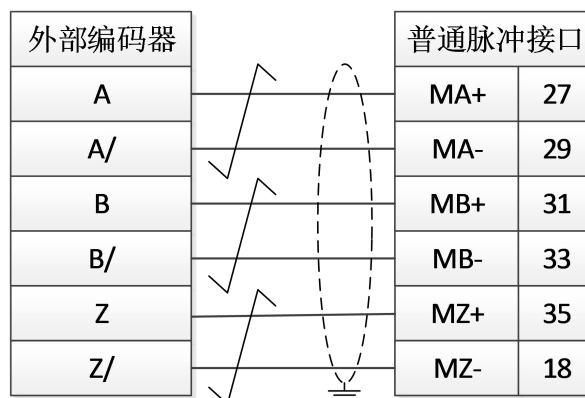
图 6-7 全闭环控制连接普通脉冲接口
