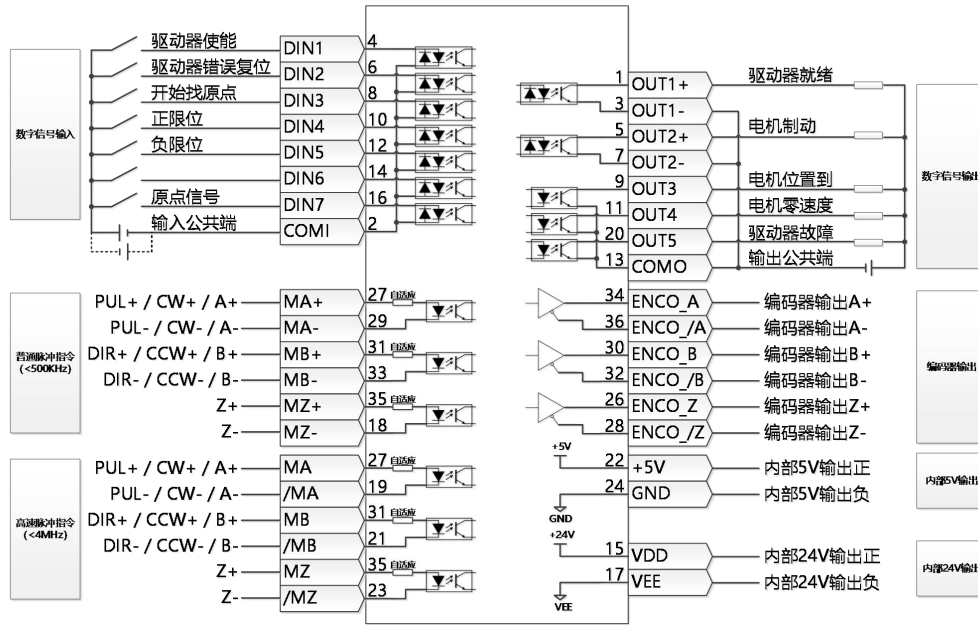
图 3-13 FD5-LA/CA 驱动器 IO 口默认定义
